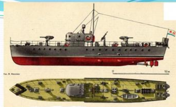
Малый охотник за подводными лодками типа «МО-4». Схема общего вида
